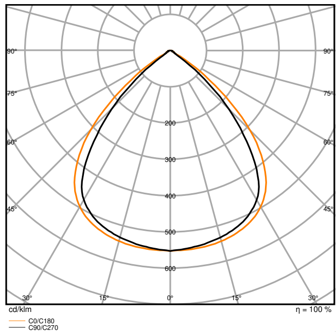
LB FLEX 1500 P 140W 840 W
