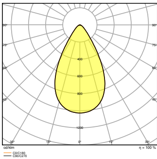
FL PFM DA 200W 3000K SYM 60 BK
