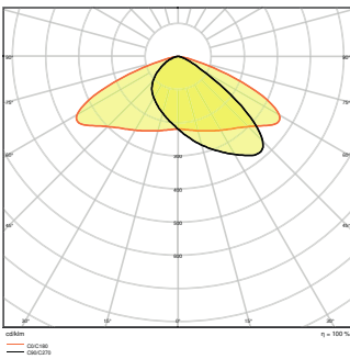
FL PFM 100W 4000K ASYM 45x140 BK
