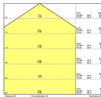
PL CMFT 625 P 28W 830 DALIVR
