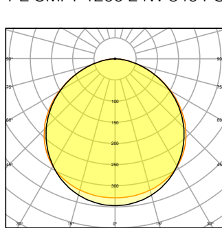
PL CMFT 1200 24W 840 PS
