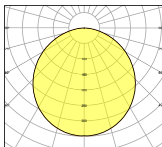
PL CMFT 625 P 28W 830 PS
