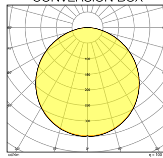
PL CMFT 625 P 24W 830 PS
