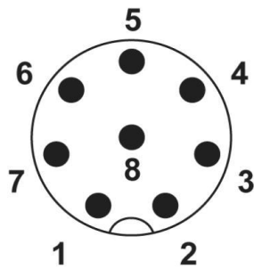
Cable
